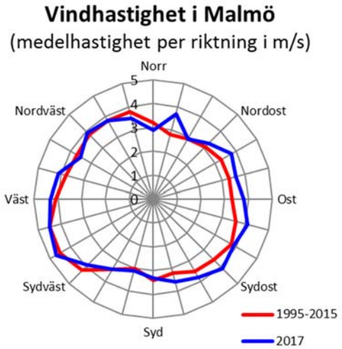
Figur 6. Medelvindhastigheten i meter per sekund för de olika vindriktningsektorerna under 2017, jämfört med medelvärdet för perioden 1995-2015.
