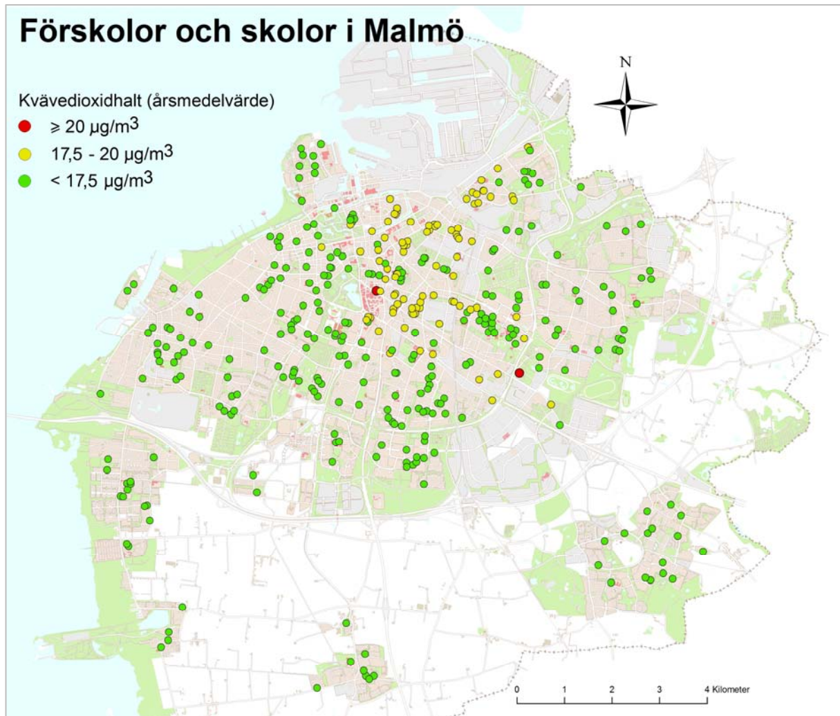
Figur 30. Beräknad kvävedioxidhalt som årsmedelvärde vid Malmös ca 450 förskole- och skolenheter. Det nationella miljömålet ”Frisk luft” ligger på 20 \mu\text{g}/\text{m}^3 . De 100 enheter som har högst halter är markerade i gult och rött.
