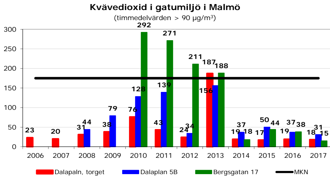
Figur 11. Antalet överskridanden av timnormen för kvävedioxid ( 90 \mu\text{g}/\text{m}^3 ) i Malmö
