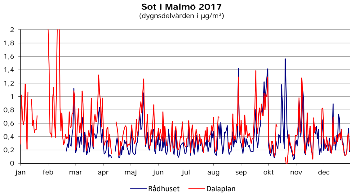
Figur 19. Dygnsprofiler för sothalter vid Dalaplan och Rådhuset under 2017.
