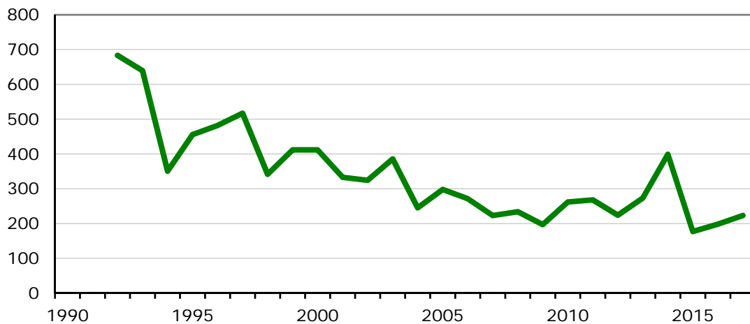
Antal timmar med vindhastighet <1 m/s i Malmö (antal timmar per år)
