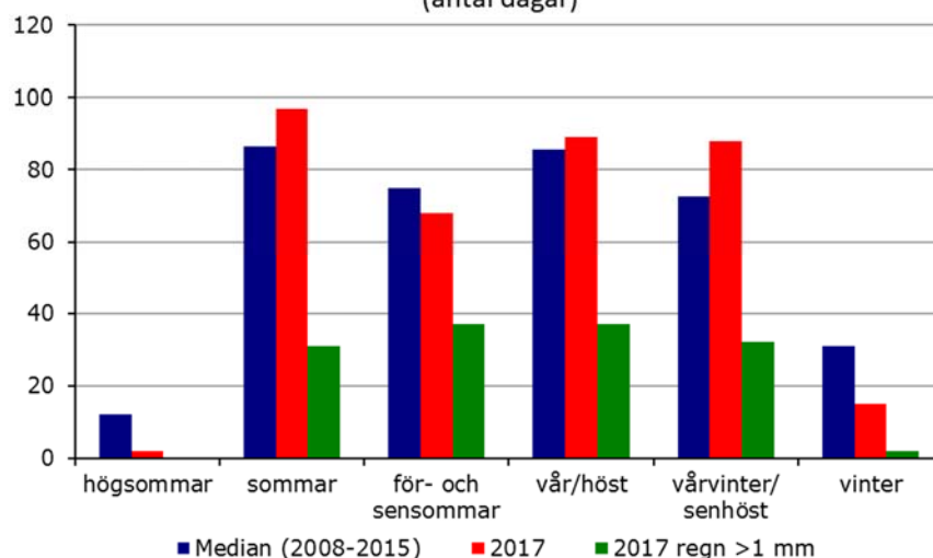
Figur 4. Fördelningen av antal dagar för sex väderkategorier under 2017.
