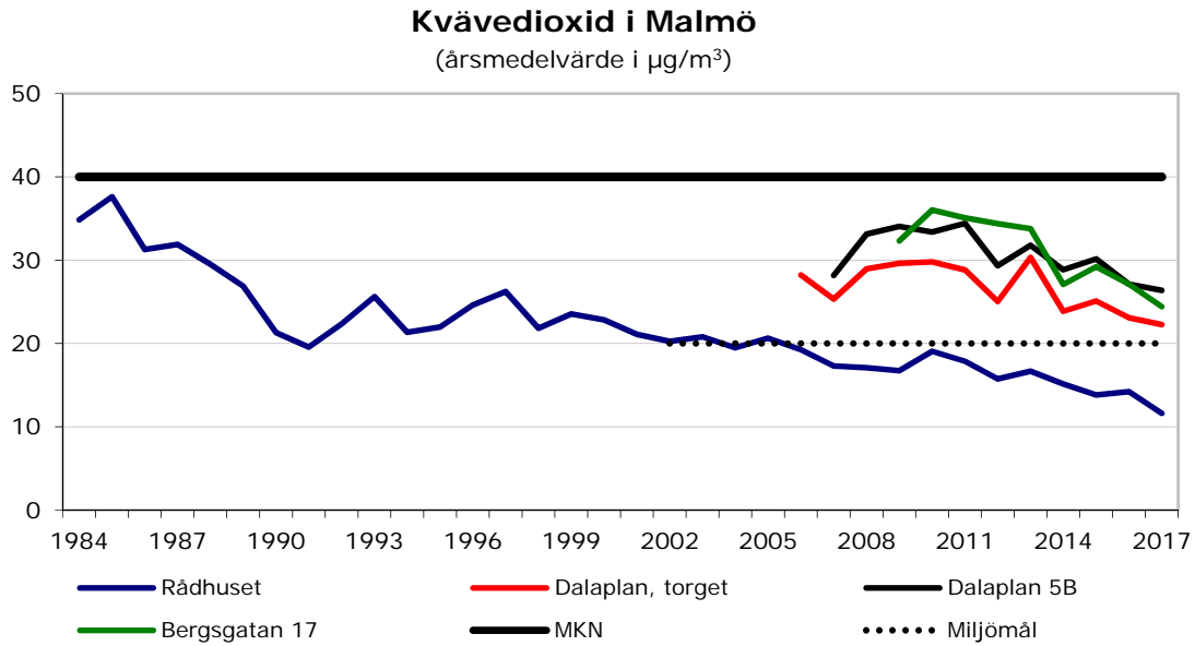
Figur 10. Kvävedioxidhalterna i Malmö som årsmedelvärden i \mu\text{g}/\text{m}^3 . Endast data från mätstationer som är aktiva 2017 presenteras.
