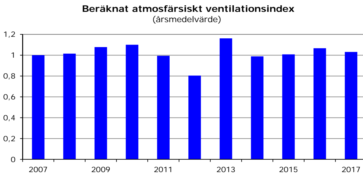
Figur 9. Atmosfäriskt ventilationsindex, mellan åren 2007 och 2017, visar vädrets inverkan på de luftföroreningar som släpps ut i Malmö.
