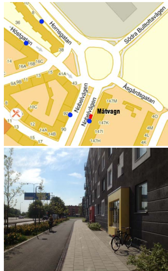
Figur 25. Nobelvägen 147K, ovan karta med mätpunkter samt nedan vy norrut mot Hornsgatan.
