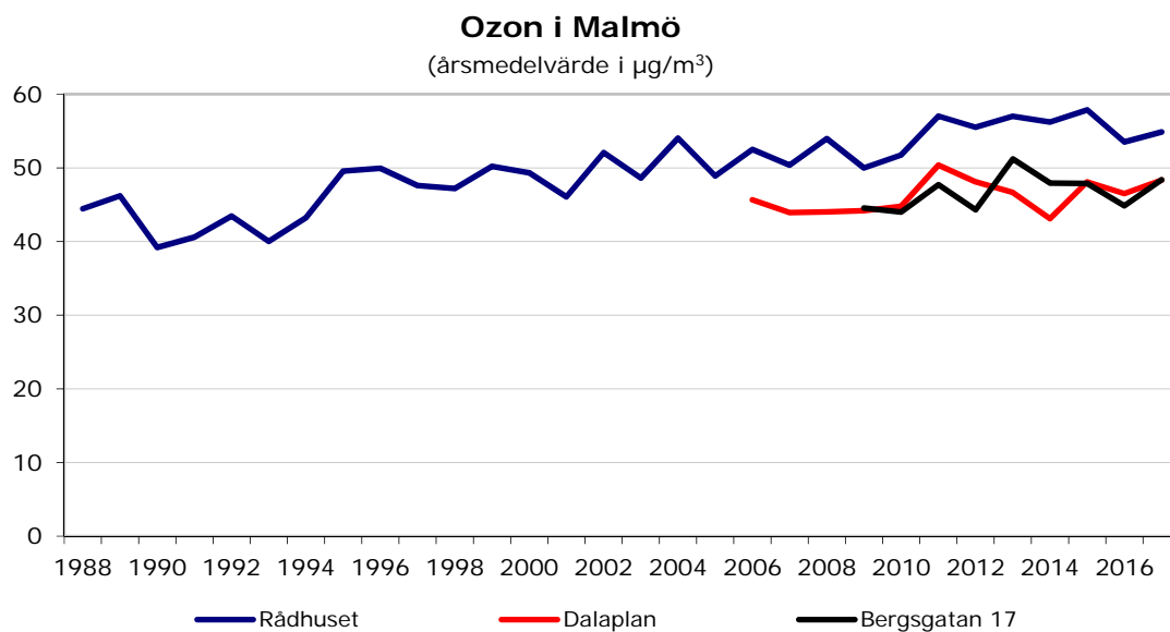
Figur 20. Ozonhalterna i Malmö som årsmedelvärden i \mu\text{g}/\text{m}^3 . Endast data från mätstationer som är aktiva idag presenteras.
