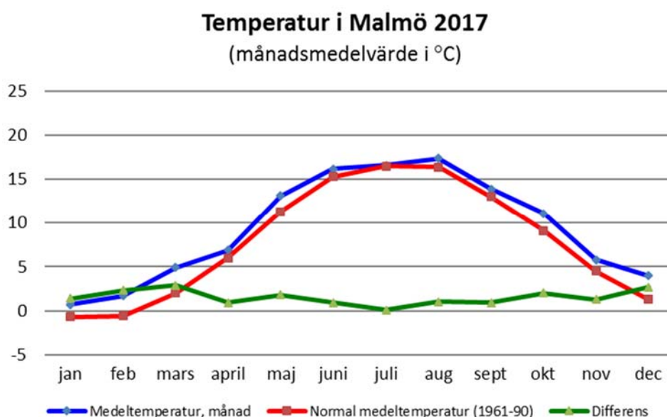
Figur 2. Månadsmedeltemperaturen i Malmö under 2017 jämfört med det av SMHI använda 30-årsmedelvärdet för 1961 - 1990. (källa: Väder och Vatten, SMHI).
