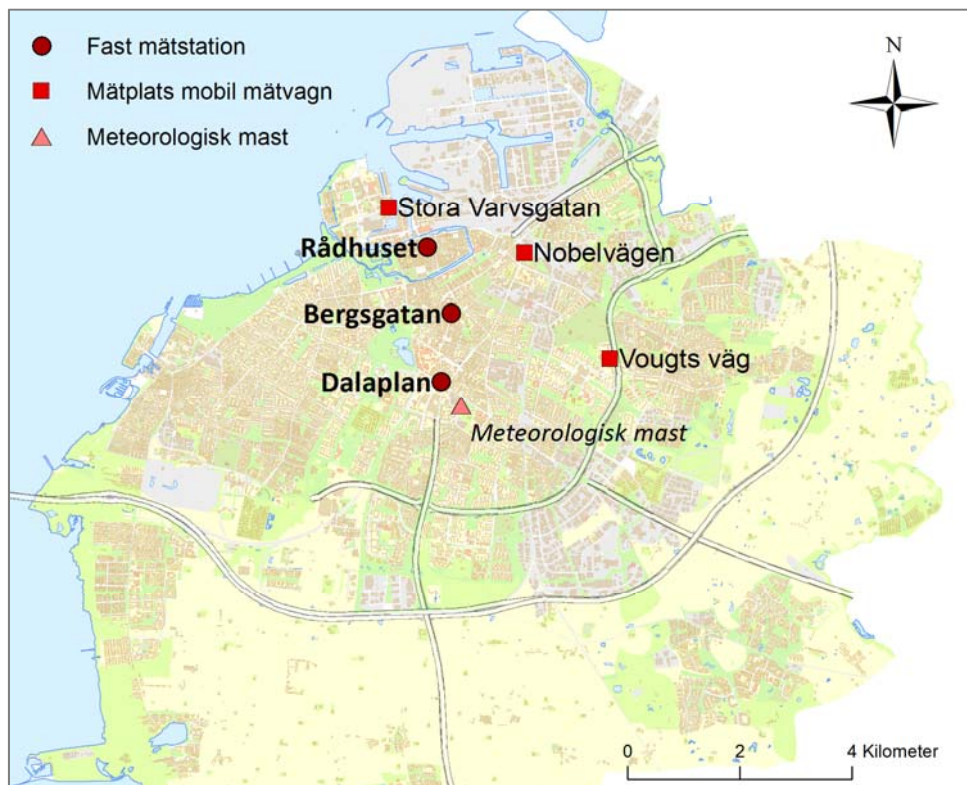
Figur 1. Karta över Malmö stads fasta och mobila mätstationer för övervakning av luftkvaliteten under 2017.
