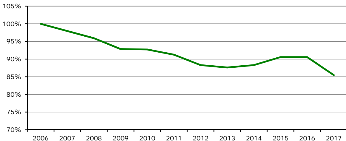
Figur 13. Utvecklingen av genomsnittlig beräknad årsmedelhalt för de 15 beräkningsplatserna i centrala Malmö för åren 2006 till 2017.
