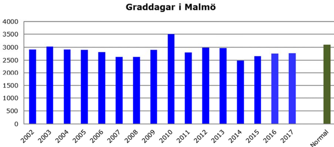
Figur 7. Groddagar utifrån temperaturmätningarna i Malmö (Heleneholm) för perioden 2002 till 2017. Antalet graddagar under ett år är summan av dygnsmedeltemperaturernas avvikelser från en referenstemperatur. Det angivna normalvärdet är medel för åren 1961-1990, där mätdata kommer från SMHI.
