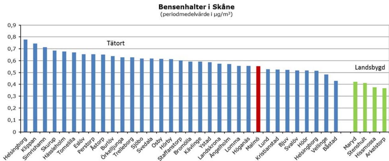
Figur 31. Bensenhalter i skånska tätorter och på bakgrundsstationer under perioden 2017-03-14 till 2017-04-19. Medelvärde av 5 separata mätningar.
