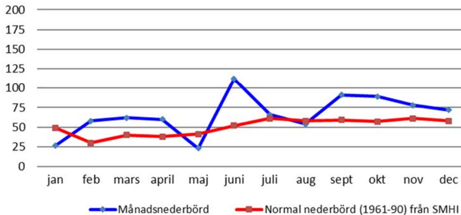
Figur 3. Månadsnederbörden i Malmö under 2017 i mm (källa: Väder och Vatten, SMHI).
