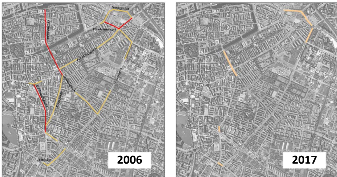
Figur 14. Gator i Malmö med risk för överskridande av miljökvalitetsnormen för kvävedioxid (gul markering, mindre än 10 % under normen) respektive överskridande (röd markering). Beräkningarna visade inte på något överskridande under 2017. Kartorna är baserade både på mätningar och beräknade lufthalter för 2006 respektive 2017.
